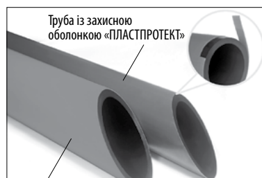
Коекструдована труба «ТВІНПЛАСТ»
